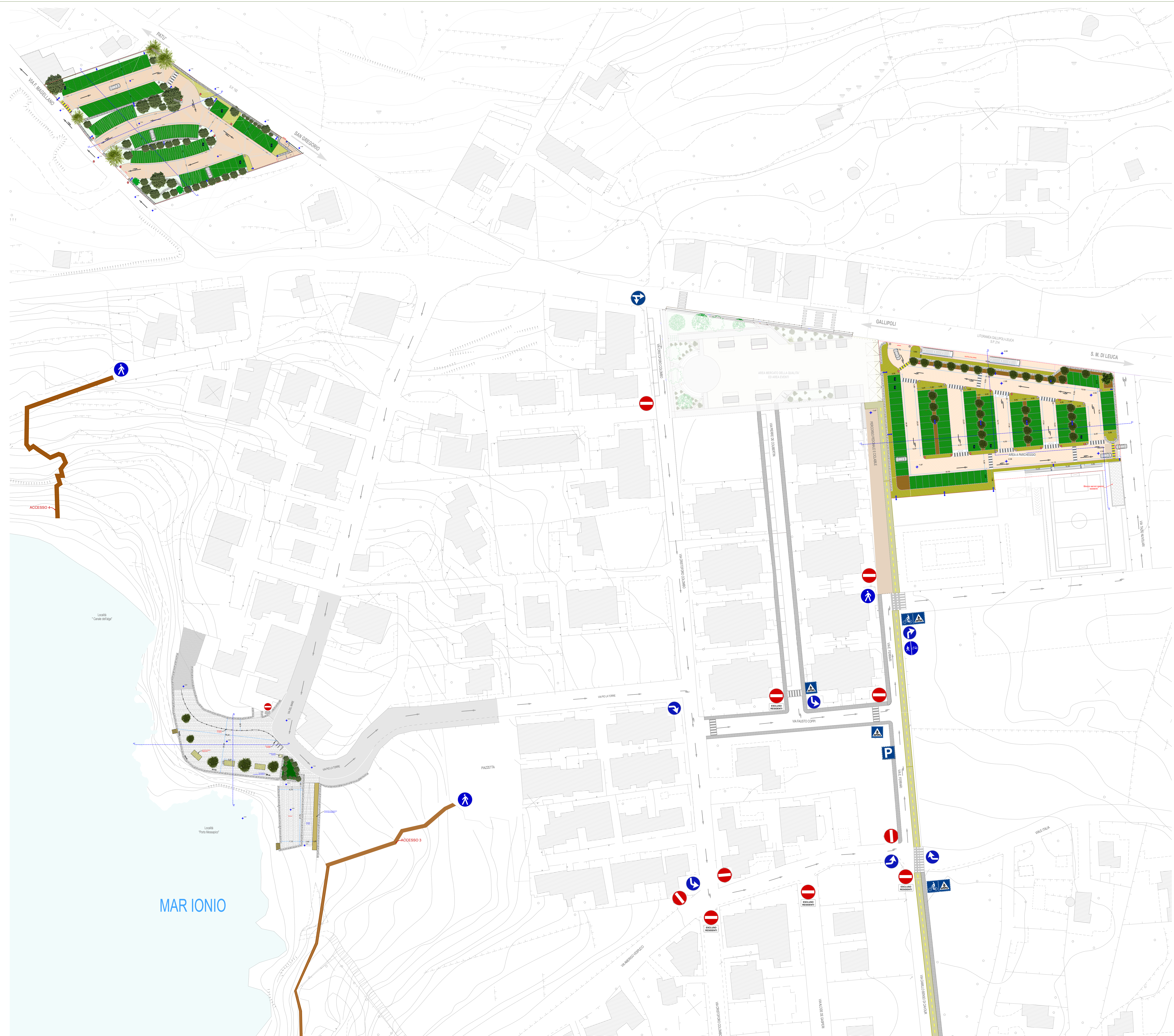
PLANIMETRIA GENERALE scala 1:500
